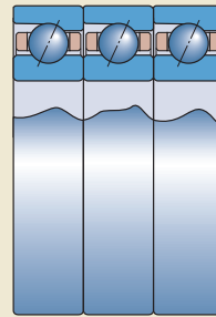
串联配置 型号后缀 TT (3T)
