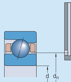
油气润滑的油喷嘴位置
