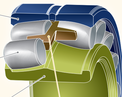
保持架
