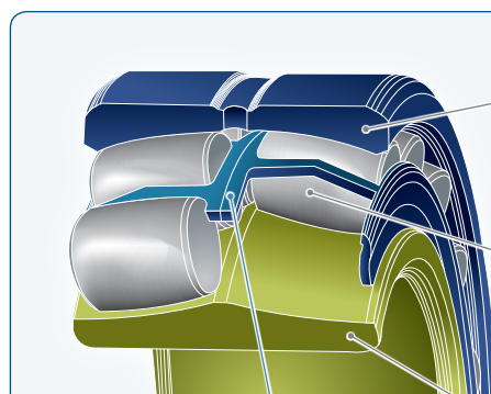
保持架
