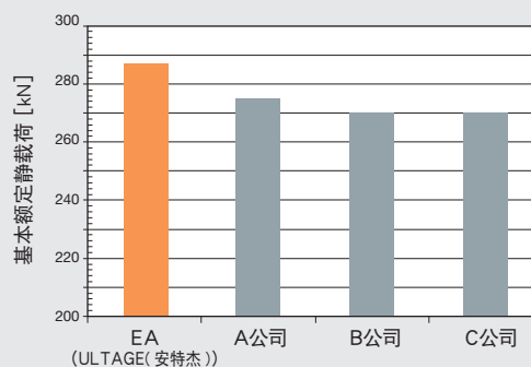
●与其他公司产品目录的基本额定静载荷( C_{or} )数值比较 22216 ( \phi 80 \times \phi 140 \times 33 )
