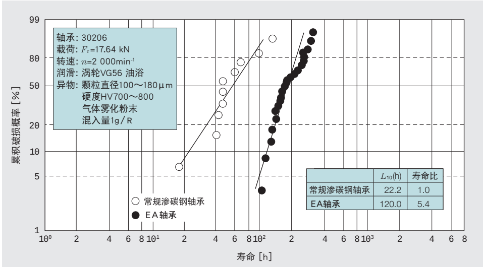
图 1 异物混入润滑下的寿命试验结果
