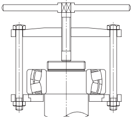
图8.53 专用拉马
