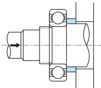
图8.50 使用压机拆卸轴承
