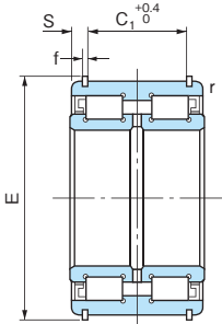
防尘盖型(E50...NR) 带止动环
