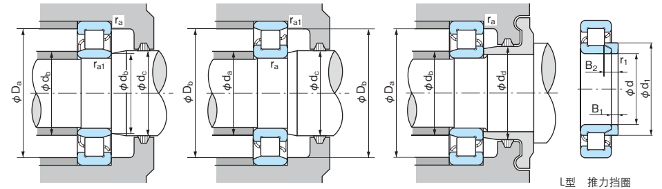
L型 推力挡圈
