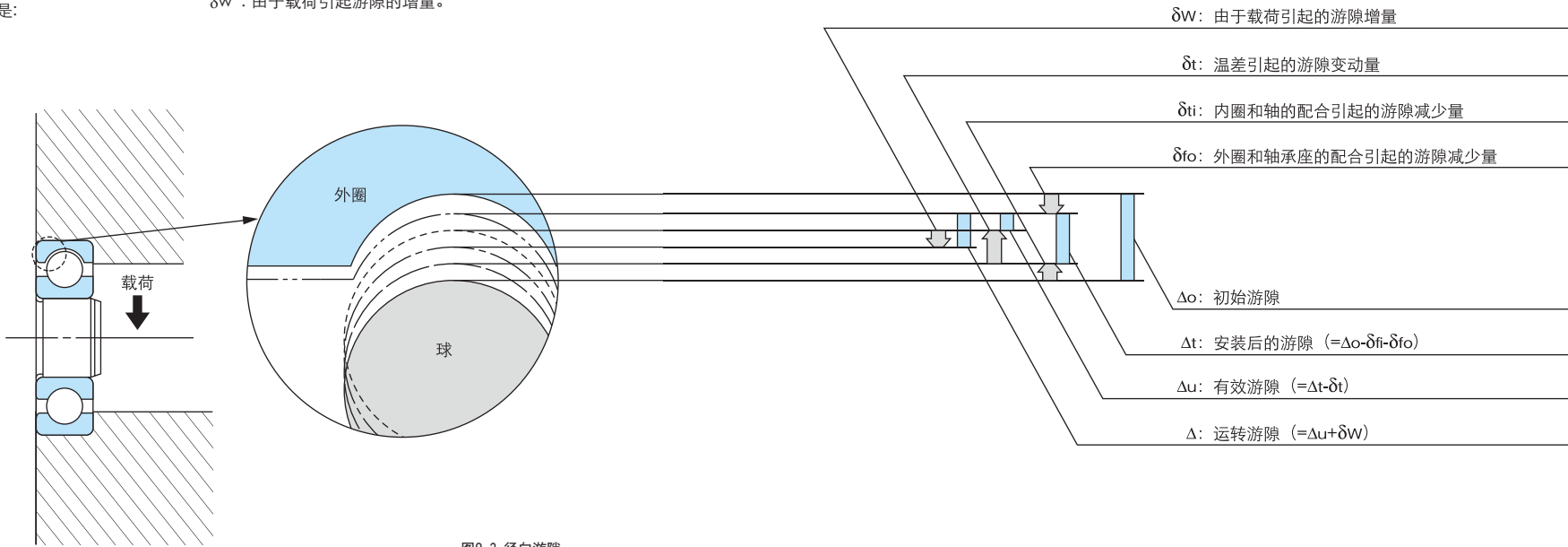
图8.3 径向游隙
