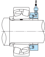
图8.45 液压螺母
