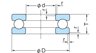
图4.3 单向推力球轴承
