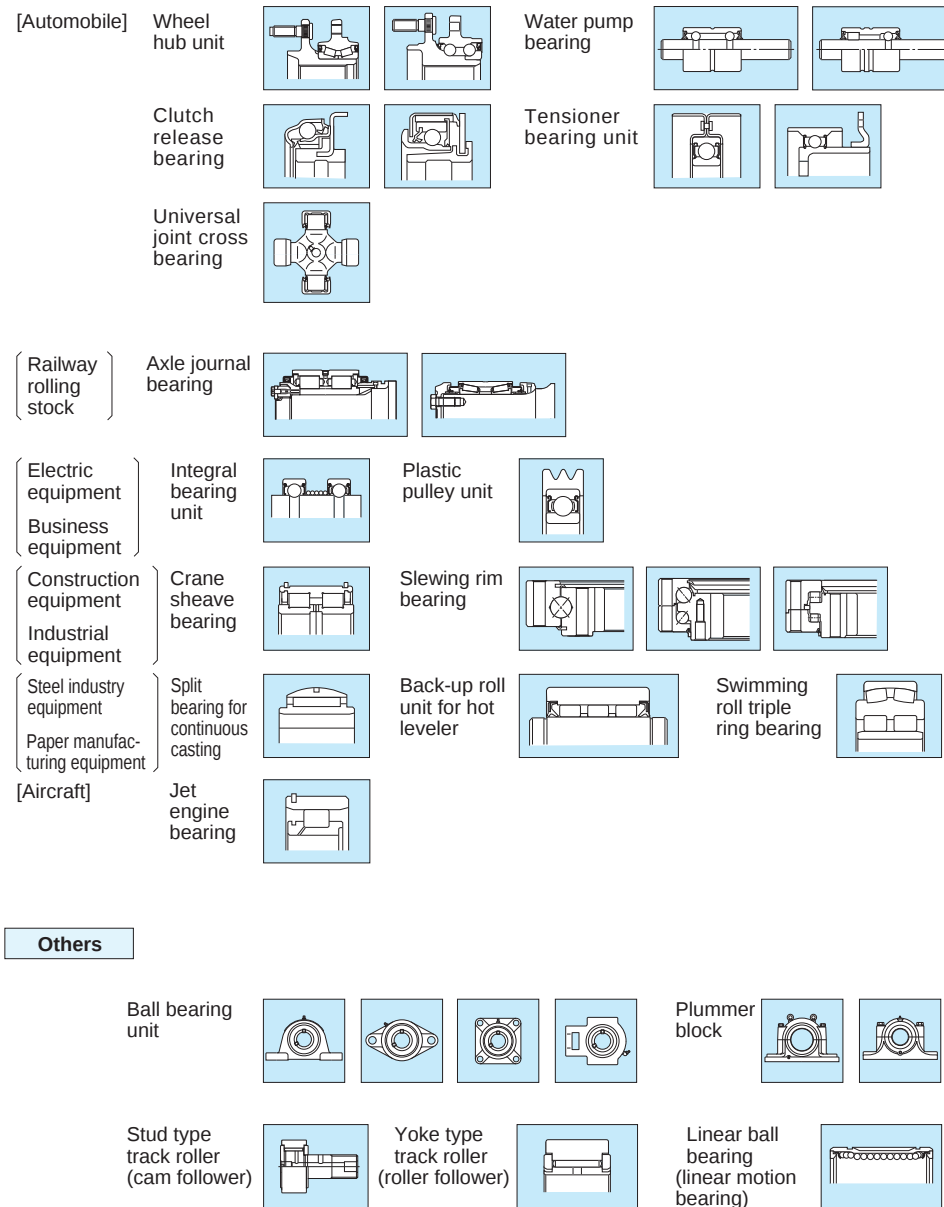
Fig. 1-2(2) Rolling bearings
