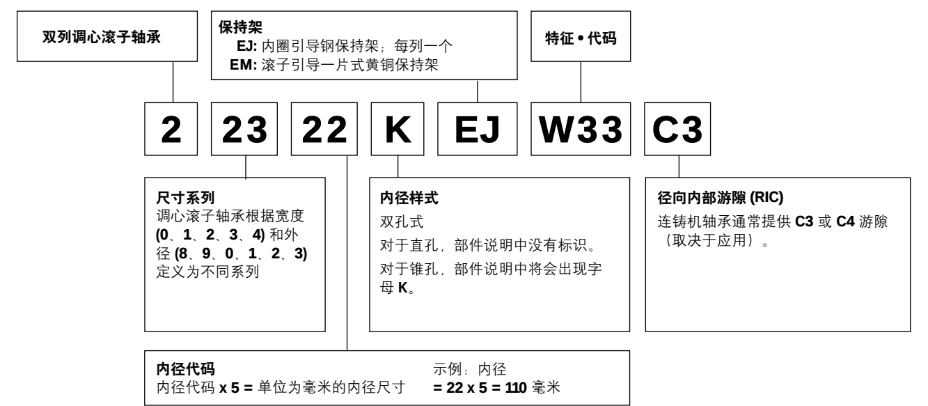
图 28. 调心滚子轴承命名规则。
