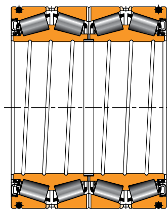
图 9. 密封辊颈轴承
