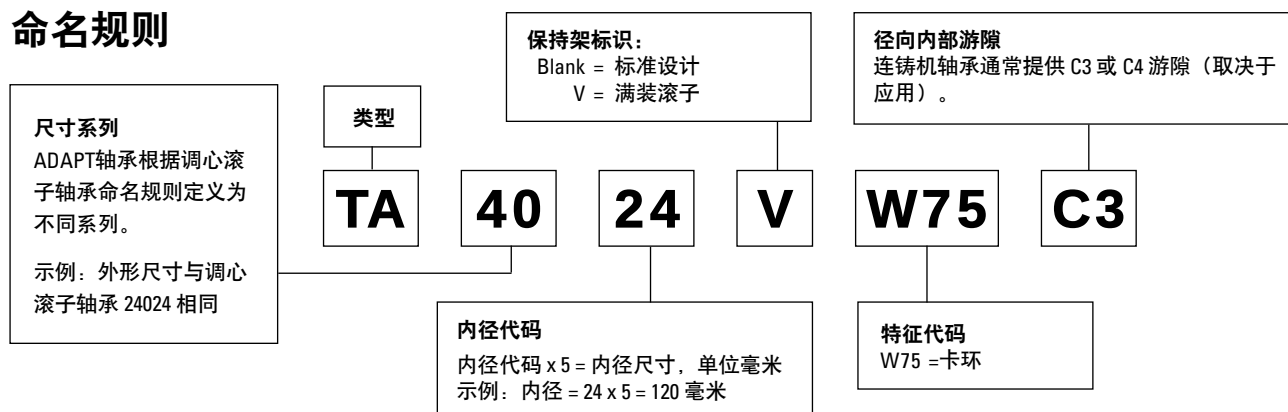
图 34. ADAPT 轴承命名规则
