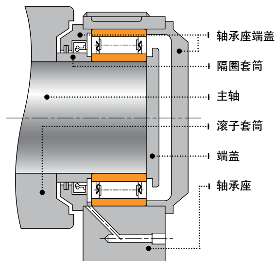
图 35. ADAPT 轴承
