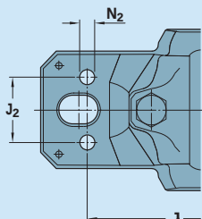
SNL.../MS2
