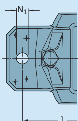
SSNLND.../MS1
