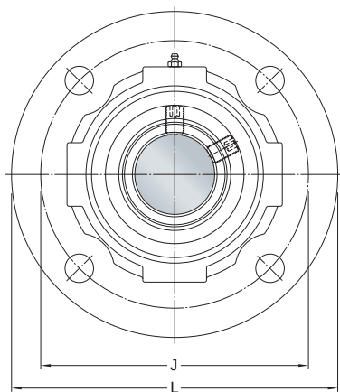
FYR
