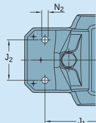
SSNLND.../MS2
