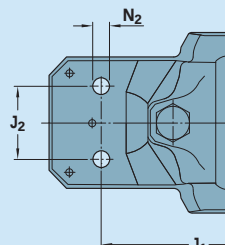
SSNLD.../MS2
