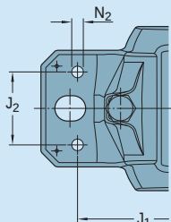
SNLN.../MS2
