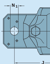
SSNLD.../MS1
