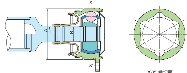
X-X' 横切面
