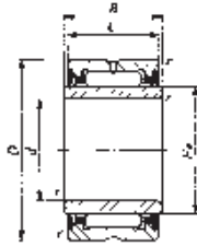
NA49...UU NA69...UU( d \leq 30 )
