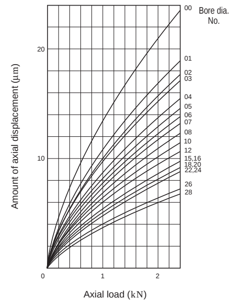
(7) 7200B (contact angle 40°)
