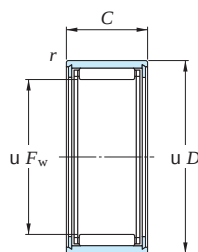
NK ( u F_w \leq 10 )
