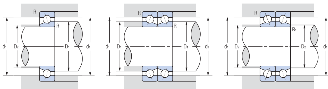
单列或者串联组配
