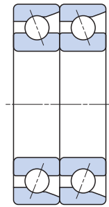
串联组配(DT)
