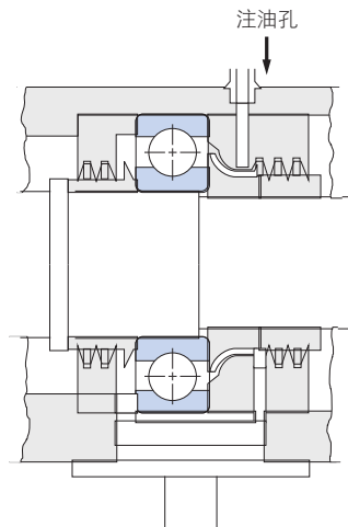
● 图6.3 甩油环喷雾器的使用例
