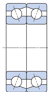
面对面组配(DF)
