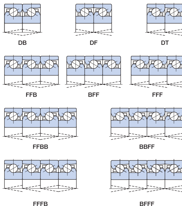
● 图4.3 自由组配轴承的组配方式与组配记号的方向 (仅限于滚珠丝杠支撑轴承TAB系列)
