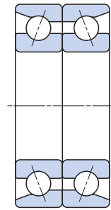
背对背组配(DB)
