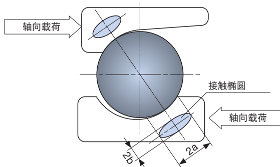
● 图2.3 接触椭圆
