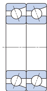
串联组配(DT)
