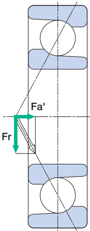
● 图2.1 角接触球轴承的轴向分力
