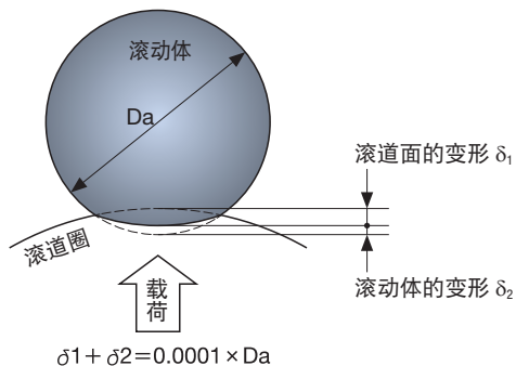
● 图2.2 永久变形量
