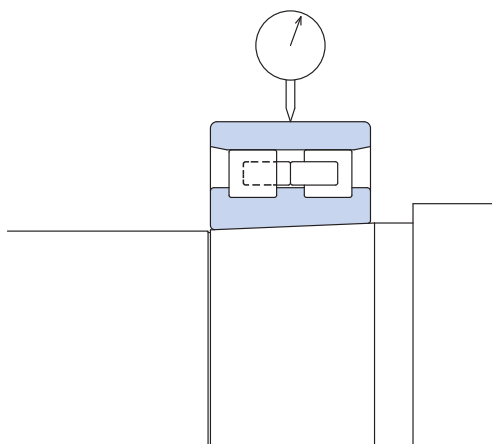
● 图9.9 径向游隙的测定
