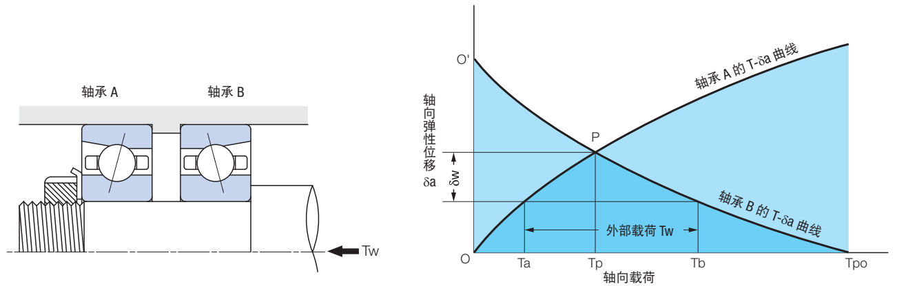
● 图5.3 定位预载荷的说明
