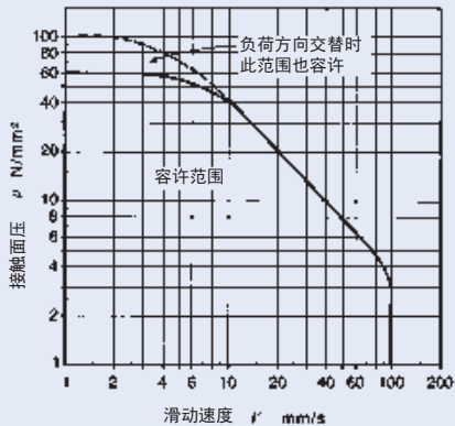
图1 加油式关节轴承的pV曲线图
