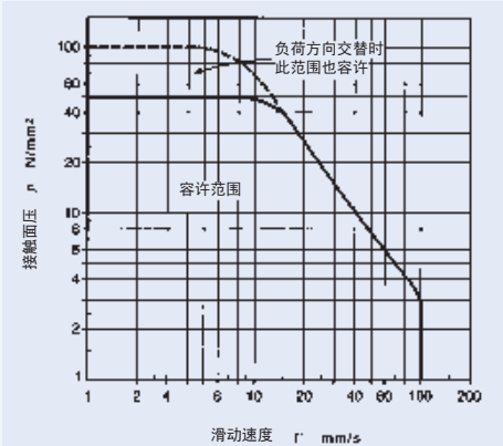
图4 不加油式关节轴承的 pV 曲线图
