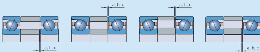
增加预载荷 (背对背)
