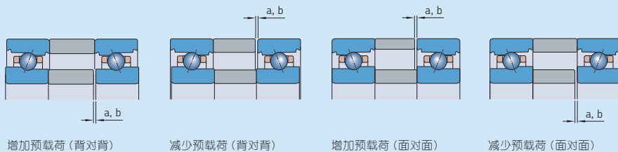
隔圈宽度减少量的指导值 - 719..B和70..B轴承系列
