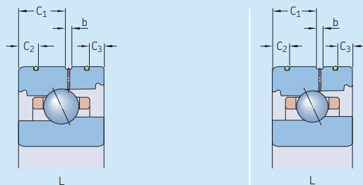
直接油气润滑的719..B和70..B轴承系列的外形尺寸
