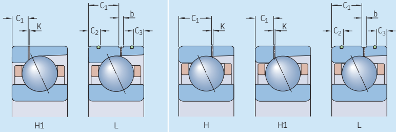
直接油气润滑的719..D和70..D轴承系列的外形尺寸
