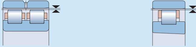
超精密圆柱滚子轴承的内部径向游隙
