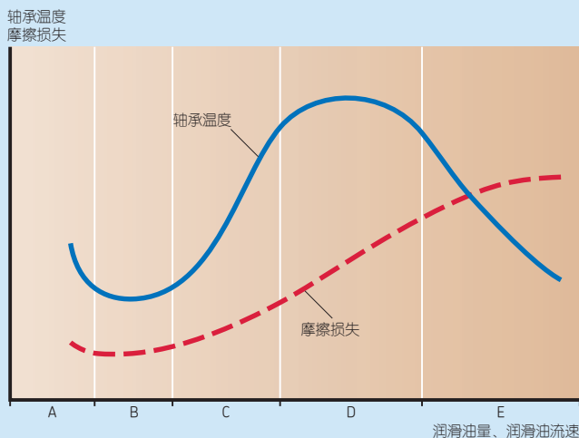
轴承温度和摩擦损失随润滑油量的变化
