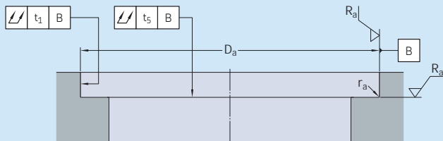
轴承座安装面的几何精度
