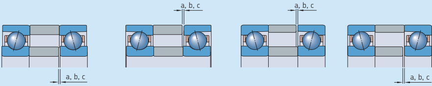
隔圈宽度减少量的指导值 - 72..D轴承系列
