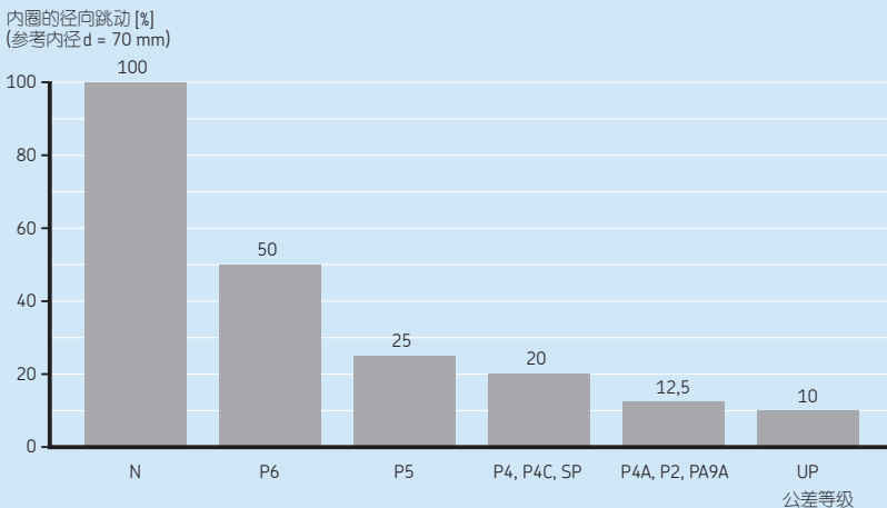
不同公差等级的相对径向跳动极限
