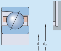
角接触球轴承喷油嘴位置
