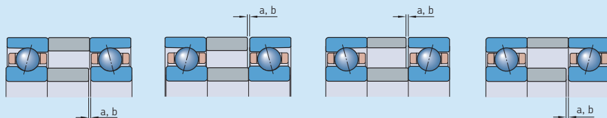
隔圈宽度减少量的指导值 - 718..D轴承系列
