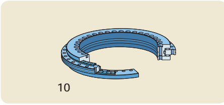
推力-向心圆柱滚子轴承 (→ 第319页) 基本设计 (NRT系列) (10)
