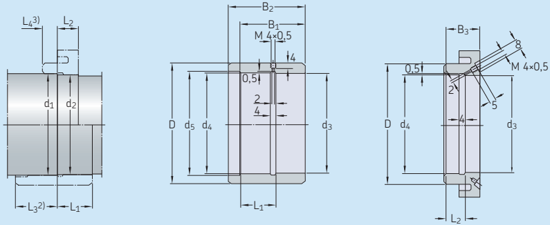
阶梯轴套及其安装面的推荐尺寸
