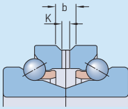
BTW..W33系列轴承环形槽和润滑孔的尺寸
