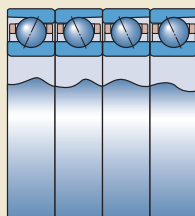
背对背+串联配置 代号后缀QBT
