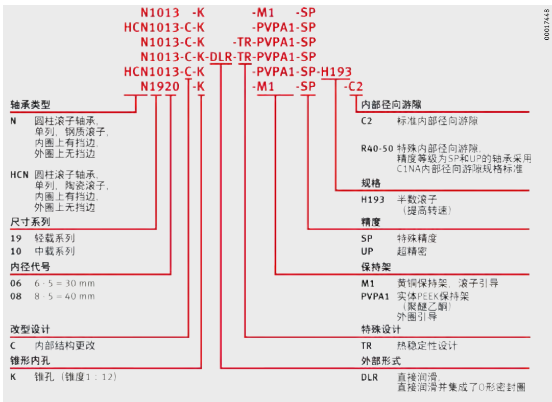
图 4 轴承型号
