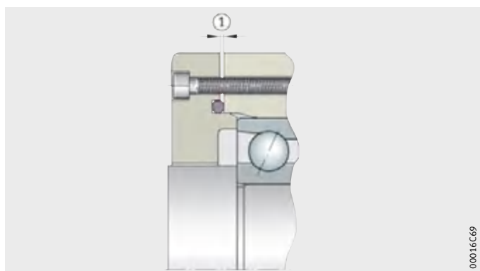
图 1 端盖匹配 (推荐)
