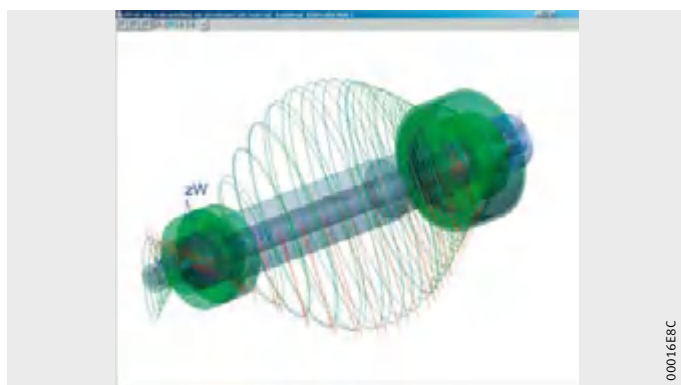
图 3 轴的变形
