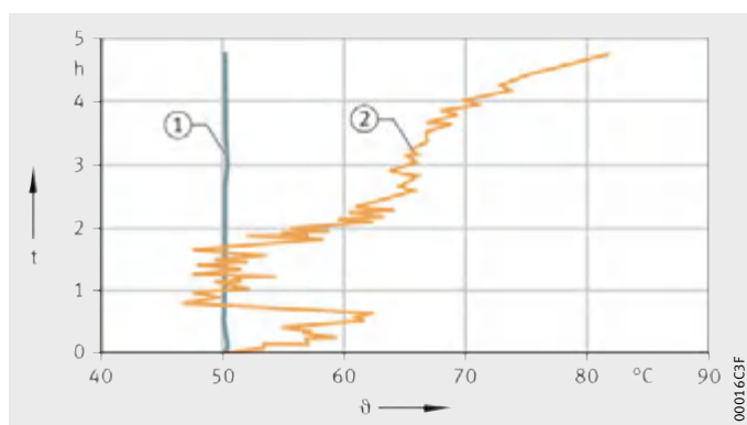
图 1 轴承温度变化
