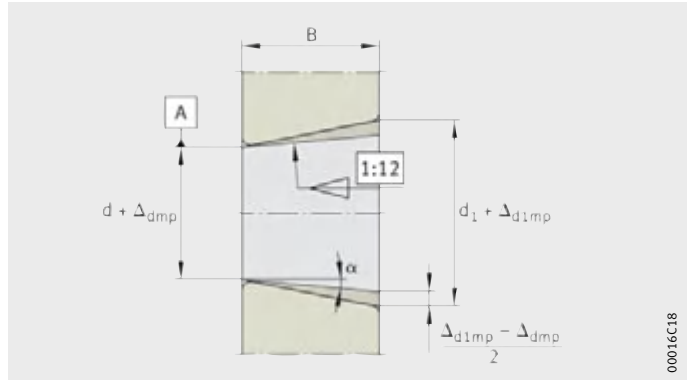
图 8 圆锥孔公差
