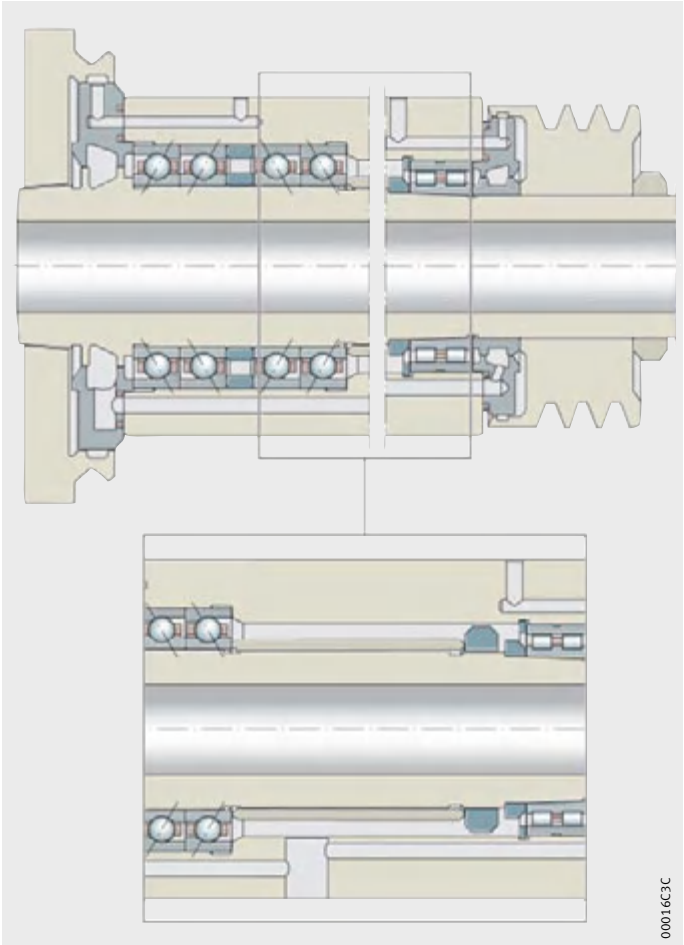
图 9 磨床主轴
