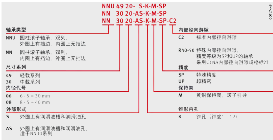
图5 轴承型号
