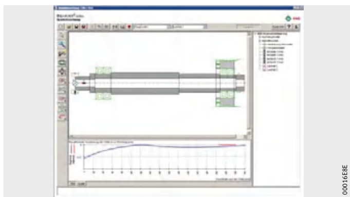
图 4 主轴上载荷分布的计算
